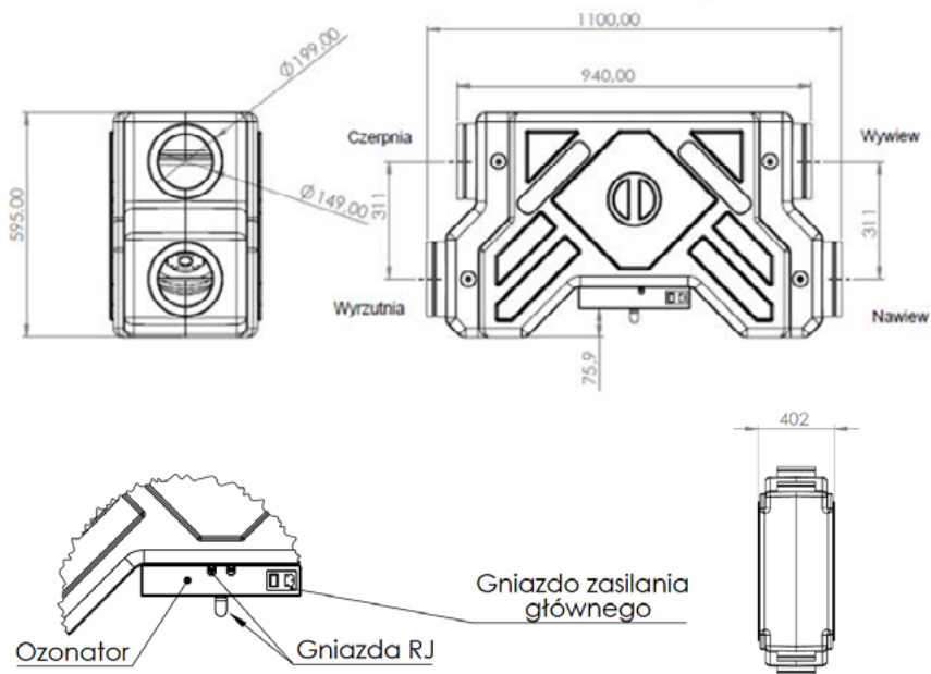
Rysunek. Wymiary nominalne centrali wentylacyjnej Matrix
