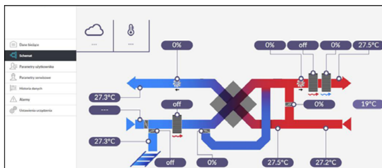
Obsługiwany schemat systemu wentylacji
