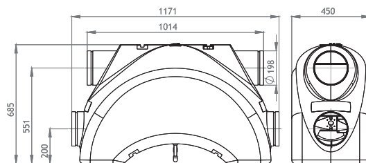
Rys. tech. Centrala rekuperacyjna LUNA 350 ECO
