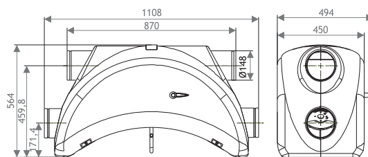
Rys. tech. Centrala rekuperacyjna LUNA 250 ECO
