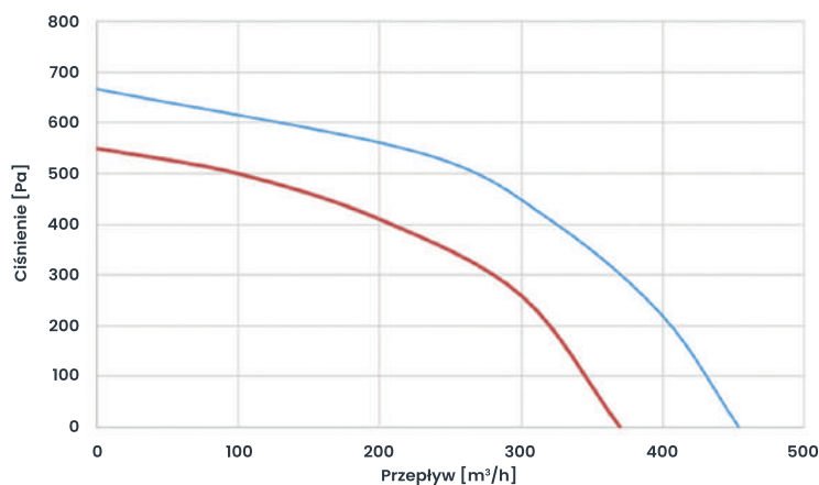
Charakterystyka przepływowa wydajności central Matrix 350, 450
