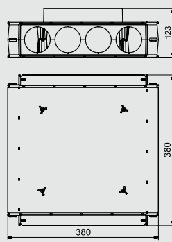
Skrzynka przelotowa Twingo
